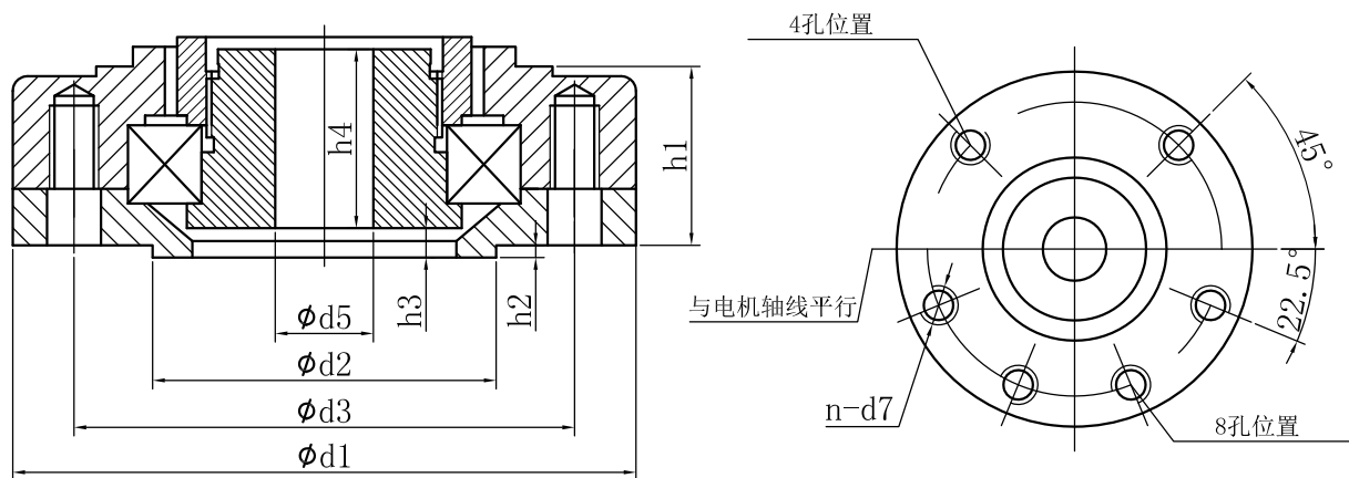
IMC系列推力型法兰型式连接尺寸
